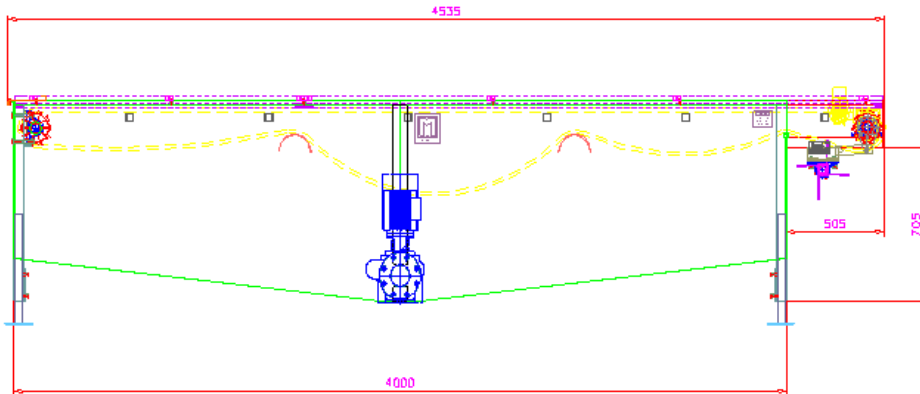
VISTA ALZADO
